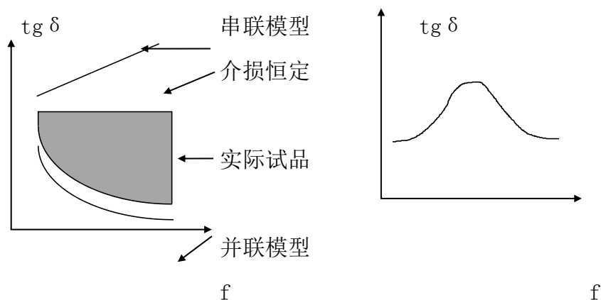
低频介损曲线(<1kHz)
