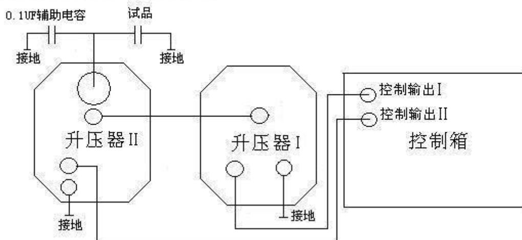
图3 (连线图)
