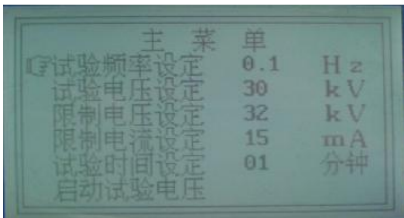
图 4 (设定界面)
