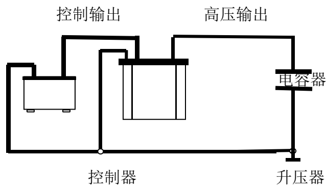
图 9 测量电容器的连线图
